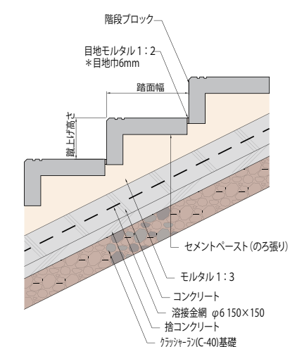
参考断面2
