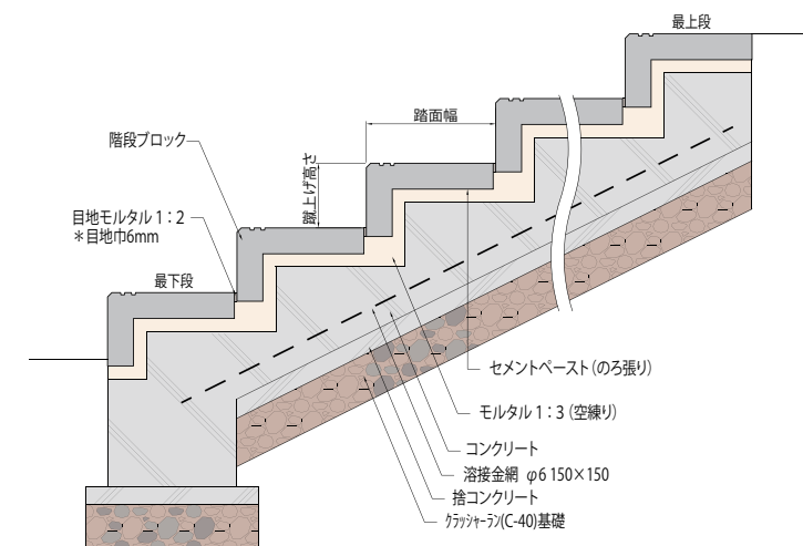
参考断面1
